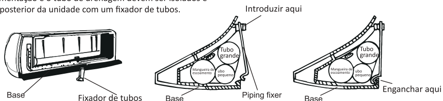
A. Introduza o fixador de tubos na ranhura.
